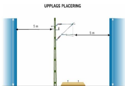
Figur 2. Exempel på tillåten placering av uppbyggnad vid elektrifierade spår.
